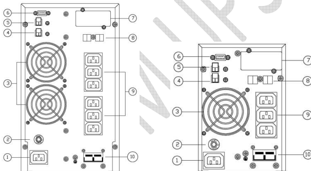
پنل پشتی دستگاه 2KVA و 3KVA باتری داخلی و بیرونی
