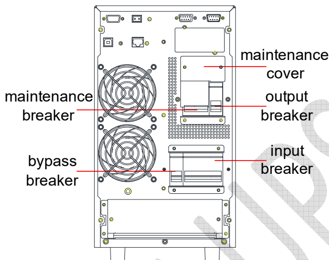
شکل ۴-۱: بای پس سرویس و نگهداری
