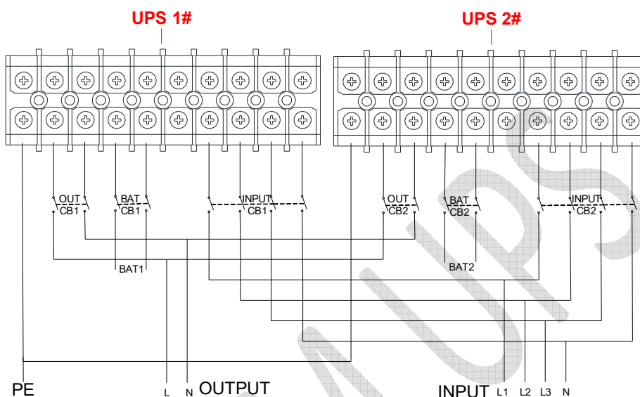
شکل ۲-۲: نحوه سیم کشی دستگاه های UPS در سیستم موازی
