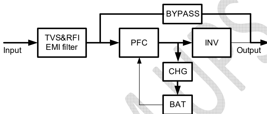
شکل ۷-۱: حالت کاری صرفه جوئی اقتصادی ECO
